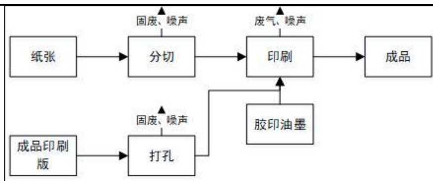
图 2-2 现有项目生产工艺流程图
