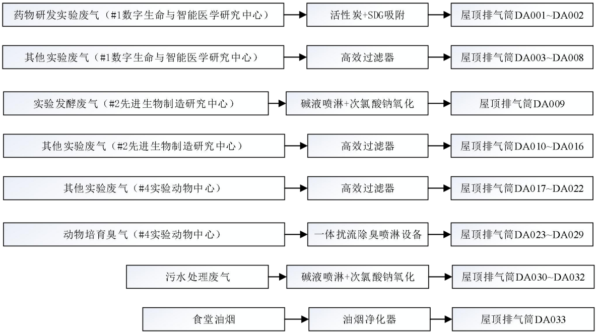
图 1-1 废气处理系统图
