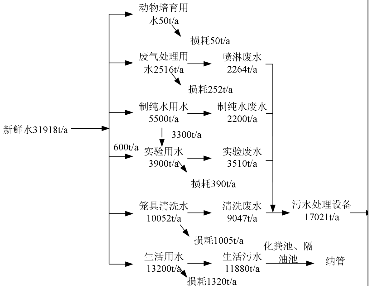
图 2-4 水平衡图
